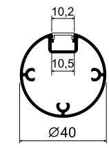
ST 01 Профиль опорный алюминиевый Длина: 6 м
