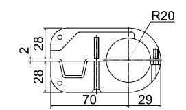
ST 05 Полкодержатель правый для полок из ЛДСП
