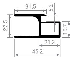
MF 33 Профиль - ручка Длина: 2,85 м
