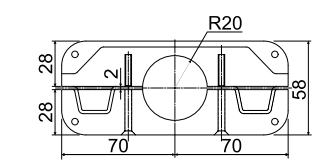
ST 06 Полкодержатель двусторонний для полок из ЛДСП
