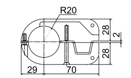
ST 04 Полкодержатель левый для полок из ЛДСП
