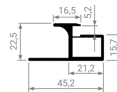
MF 34 Профиль - ручка Длина: 5,5 м
