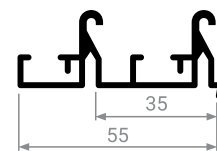
MS 62 Направляющая верхняя Длина: 5,8 м
