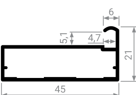
MZ 09 Профиль фасадный Длина: 6 м
