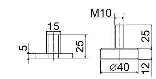
ST 02 Крепление к полу
